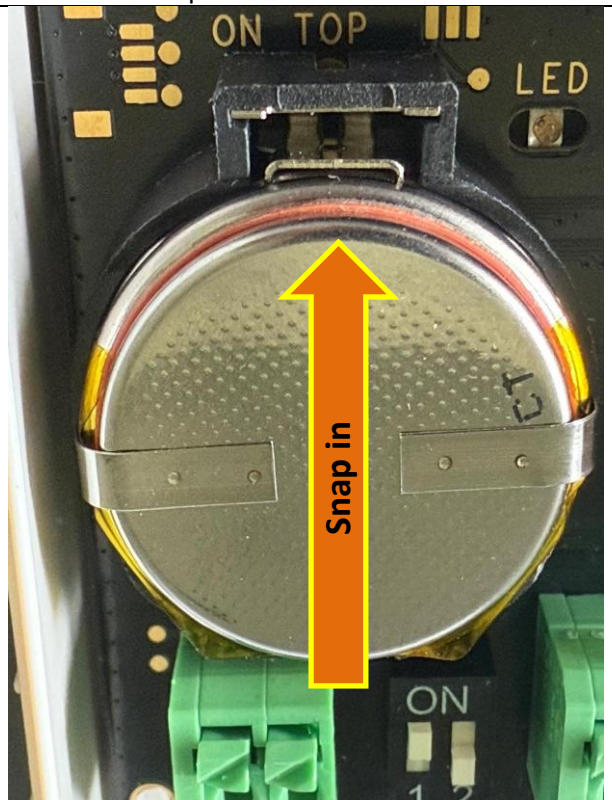
Batterij eerst aan de kant van de gele folie plaatsen en dan indrukken zodat de clip de batterij vastzet.
