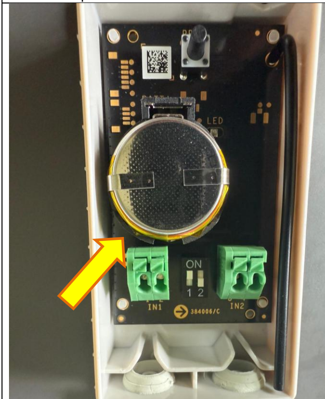
Batterij eerst aan de kant van de gele folie plaatsen en dan indrukken zodat de clip de batterij vastzet.
